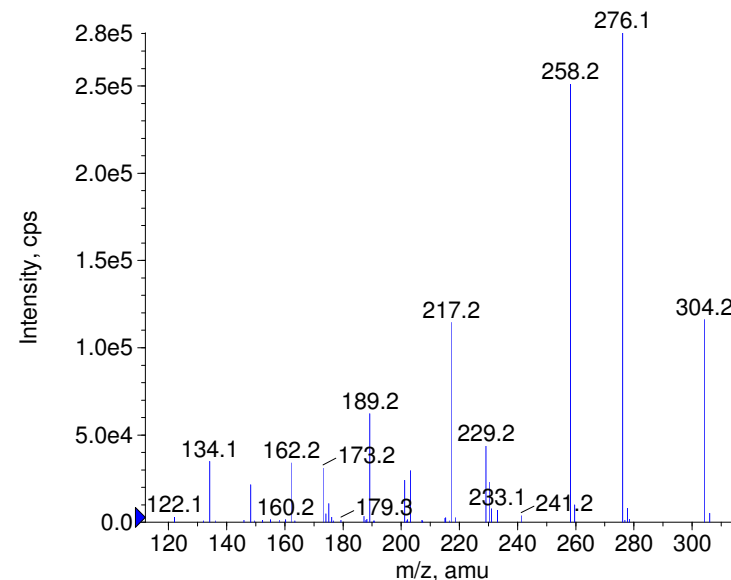
+ Flumazenil Prec(304.0) CE(99.0) RT(0.8)
