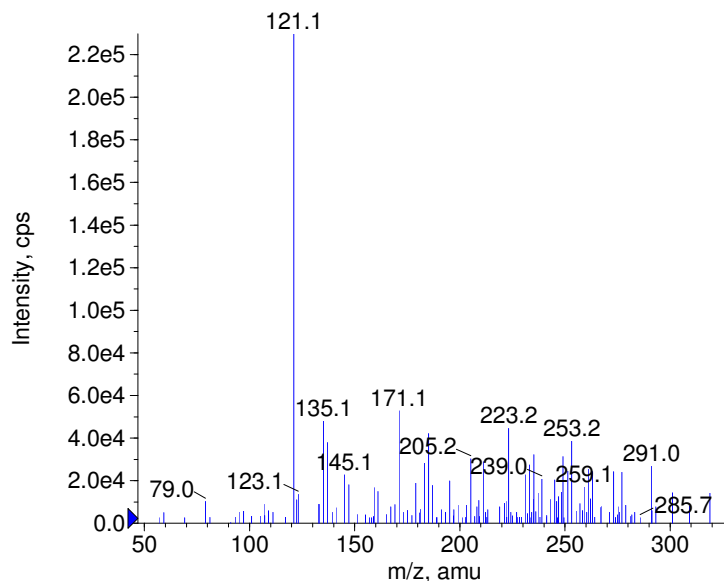
+ Fluocinonide Prec(495.0) CE(50.0) RT(0.9)
