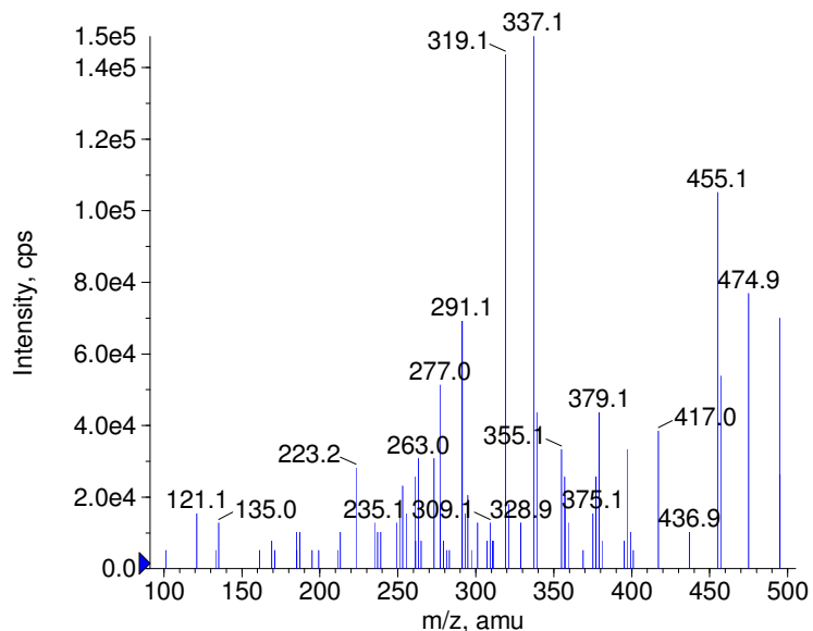
+ Fluocinonide Prec(495.0) CE(50.0) RT(0.9)
