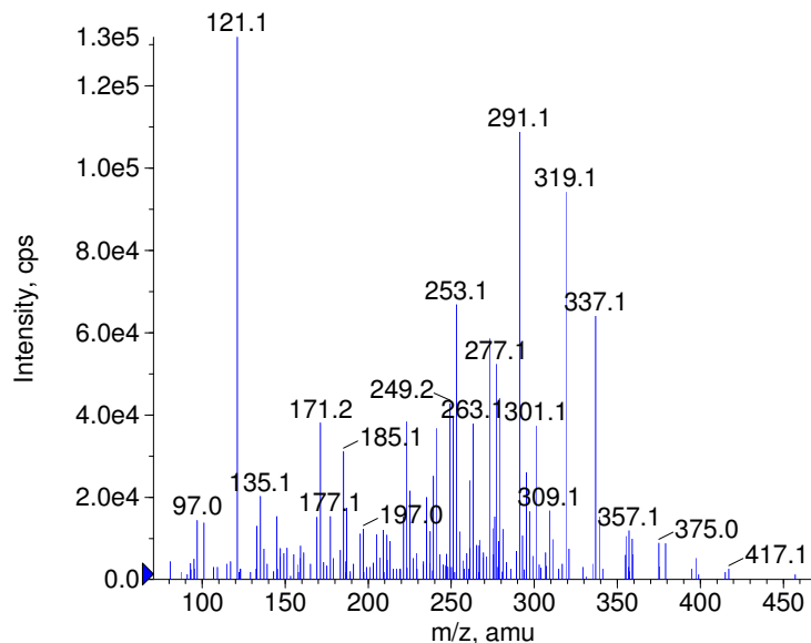
+ Fluocinonide Prec(495.0) CE(99.0) RT(0.9)
