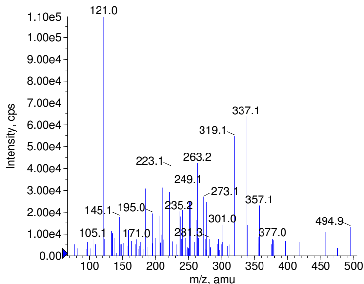
+ Fluocinonide Prec(495.0) CE(99.0) RT(0.9)
