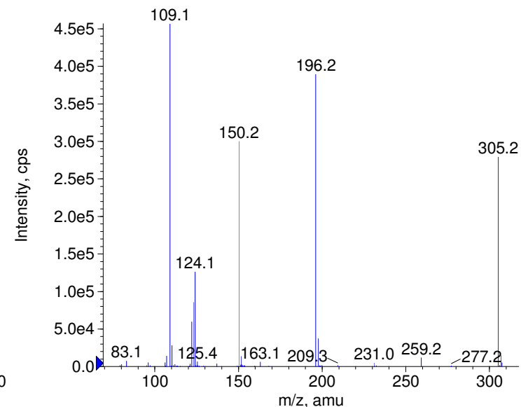
+ Flupirtine Prec(305.0) CE(99.0) RT(0.8)
