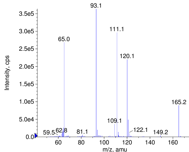
+ Formetanate Prec(222.0) CE(50.0) RT(0.8)
