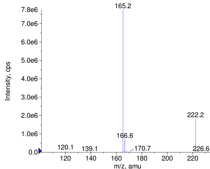
+ Formetanate Prec(222.0) CE(50.0) RT(0.8)
