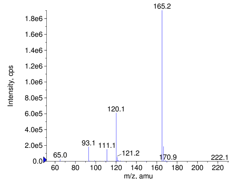
+ Formetanate Prec(222.0) CE(99.0) RT(0.9)
