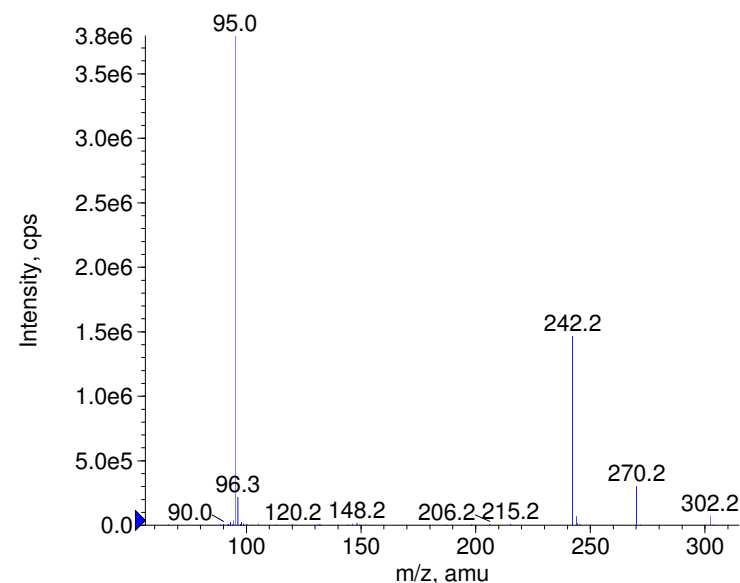
+ Furalaxyl Prec(302.0) CE(99.0) RT(1.2)
