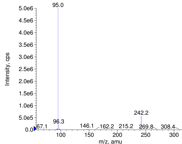
+ Furalaxyl Prec(302.0) CE(99.0) RT(1.2)
