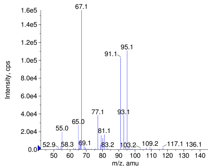
■ + Gabapentin Prec(172.0) CE(50.0) RT(0.8)
