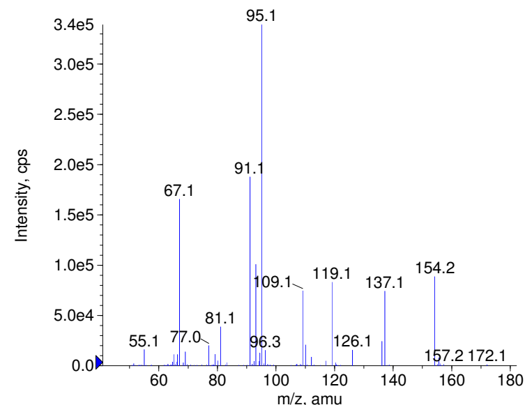
■ + Gabapentin Prec(172.0) CE(99.0) RT(0.8)
