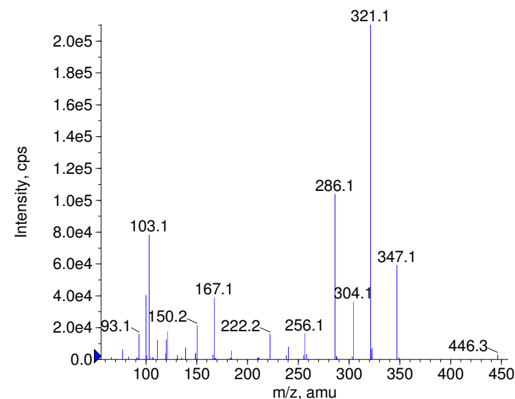
+ Glipizide Prec(446.0) CE(99.0) RT(0.8)
