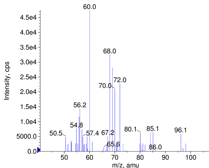
■ + Glucosamine Prec(180.0) CE(50.0) RT(0.9)
