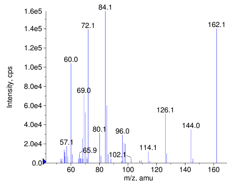
■ + Glucosamine Prec(180.0) CE(99.0) RT(0.9)
