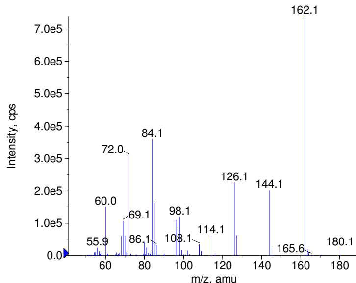
■ + Glucosamine Prec(180.0) CE(50.0) RT(0.9)
