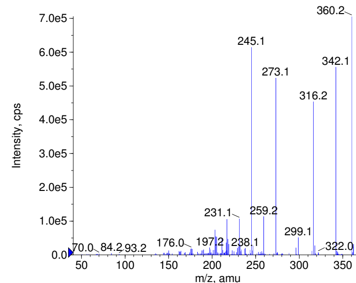
+ Grepafloxacin Prec(360.0) CE(99.0) RT(0.9)
