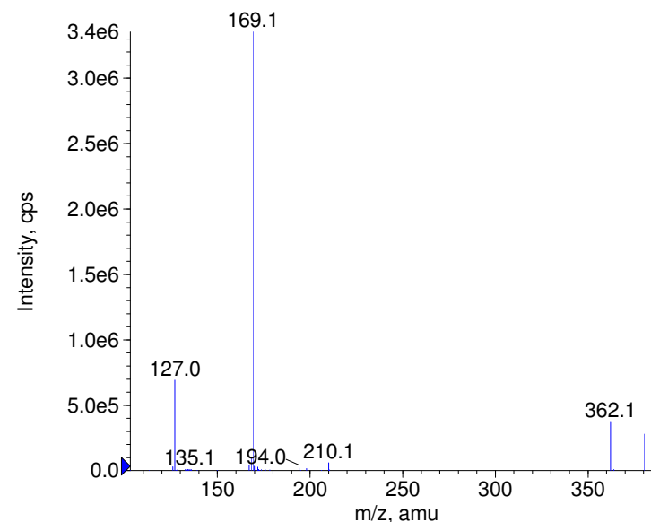
■ + Haloperidol-D4 Prec(380.0) CE(99.0) RT(0.9)
