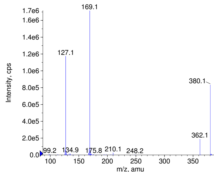
■ + Haloperidol-D4 Prec(380.0) CE(99.0) RT(0.9)
