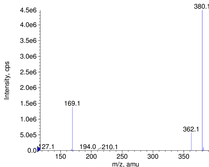
■ + Haloperidol-D4 Prec(380.0) CE(50.0) RT(0.9)
