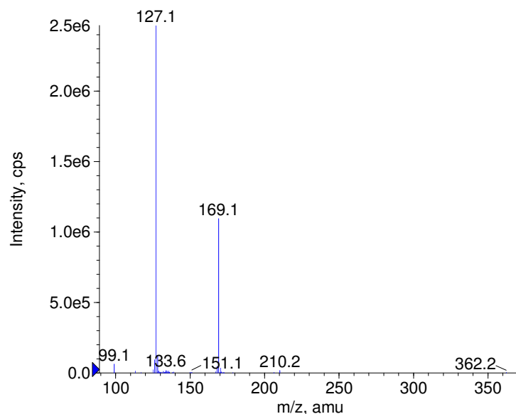
■ + Haloperidol-D4 Prec(380.0) CE(50.0) RT(0.9)
