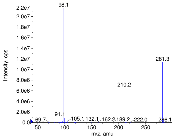
+ Histapyrrodine Prec(281.0) CE(50.0) RT(0.9)
