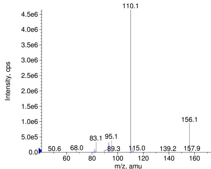
+ Histidine Prec(156.0) CE(50.0) RT(0.9)
