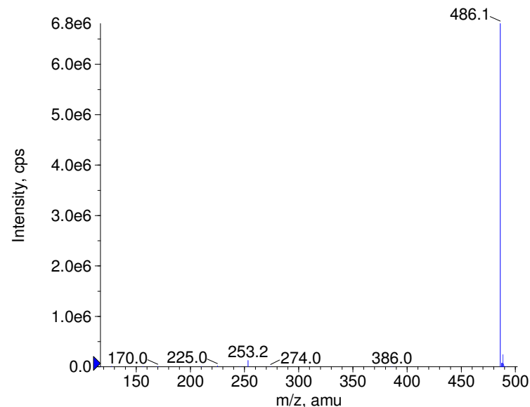
+ Imiclozapine Prec(486.0) CE(50.0) RT(1.0)
