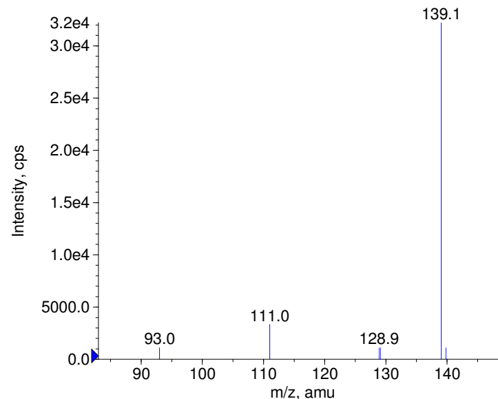
+ Indomethacin Prec(358.0) CE(50.0) RT(0.8)
