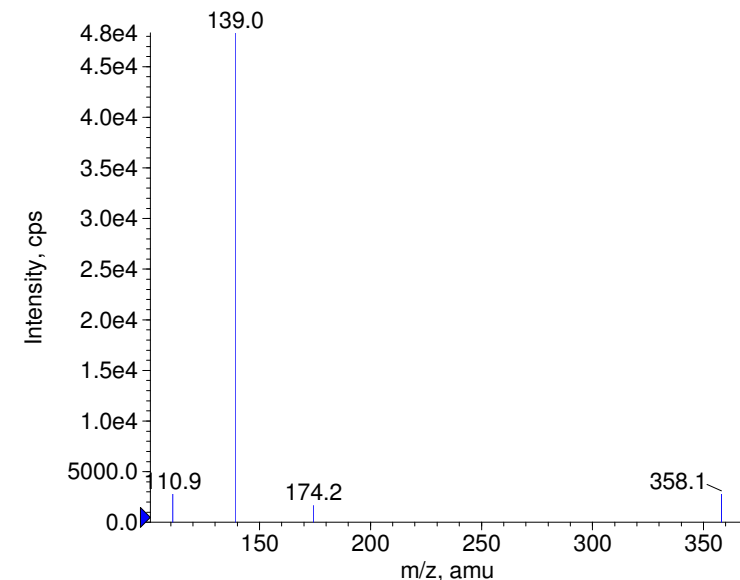
+ Indomethacin Prec(358.0) CE(99.0) RT(0.8)
