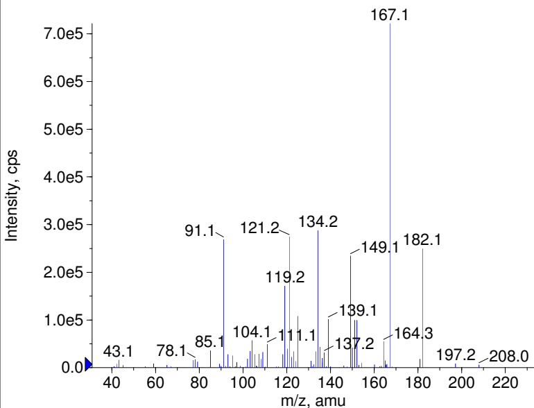
+ 2C-T-4 Prec(256.0) CE(50.0) RT(0.4)
