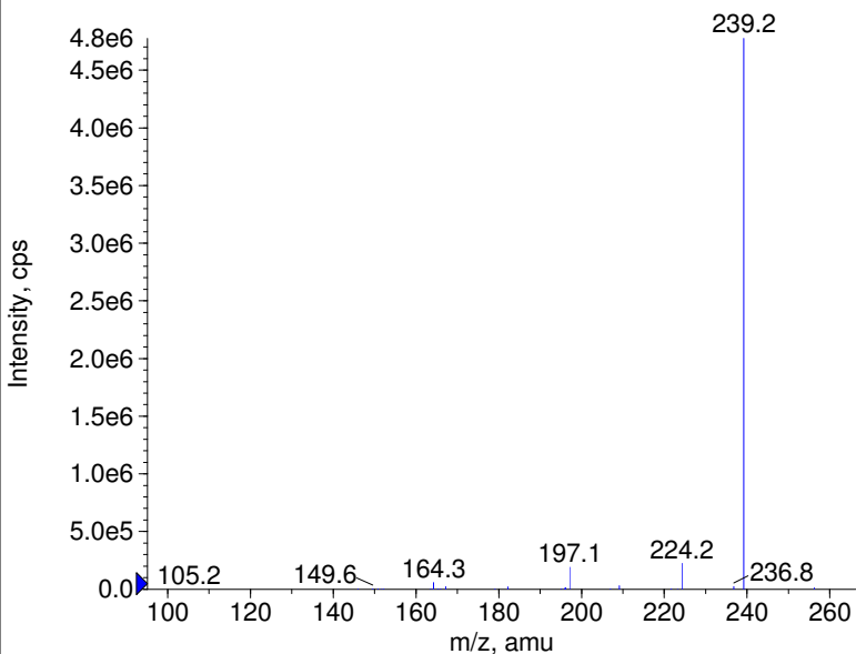
+ 2C-T-7 Prec(256.0) CE(50.0) RT(0.4)
