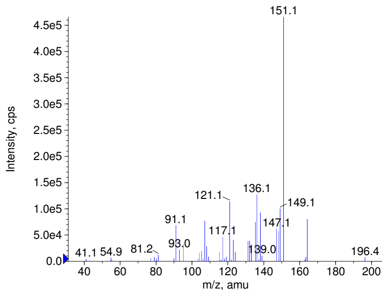
+ 3,4-DMA Prec(196.0) CE(35.0) RT(0.3)
