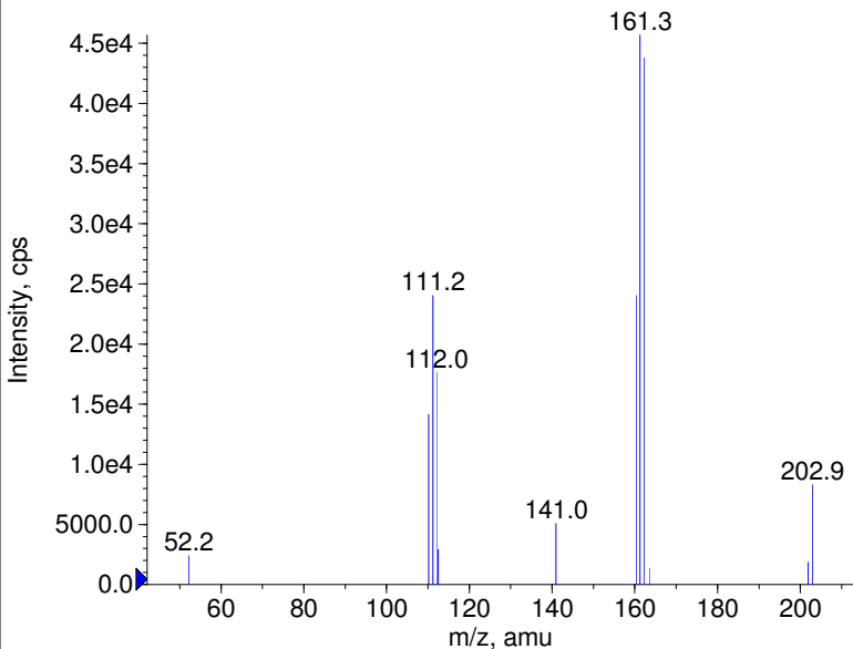
+ D10-Fenfluramin Prec(243.0) CE(50.0) RT(0.4)
