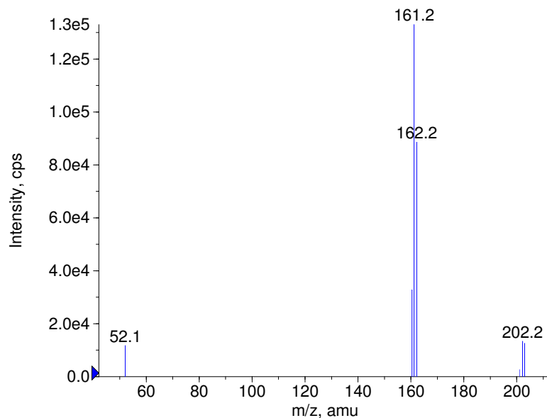
+ D10-Fenfluramin Prec(243.0) CE(35.0) RT(0.4)
