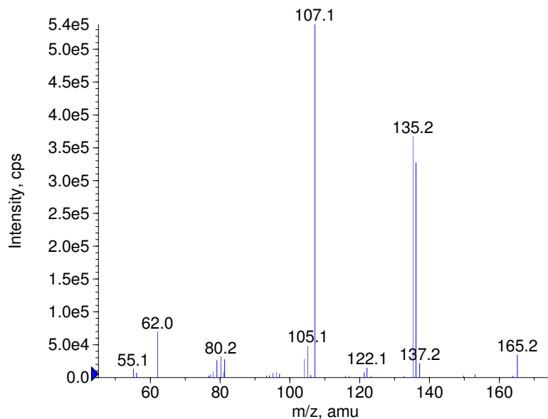
+ D5-MDMA Prec(199.0) CE(35.0) RT(0.3)
