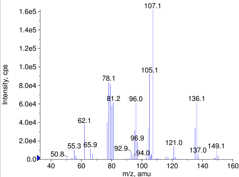
+ D5-MDMA Prec(199.0) CE(50.0) RT(0.4)
