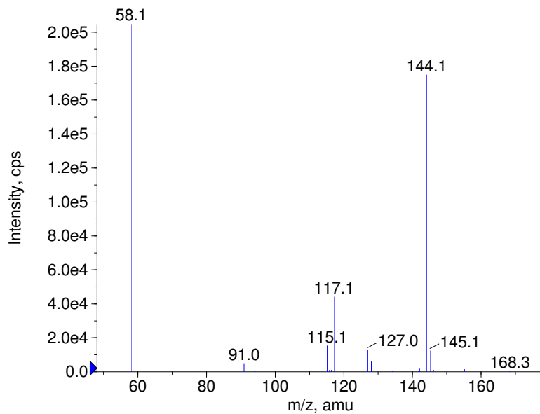
■ + DMT Prec(189.0) CE(35.0) RT(0.3)
