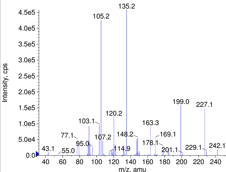
■ + DOB Prec(274.0) CE(50.0) RT(0.3)
