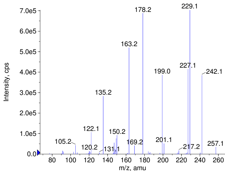
■ + DOB Prec(274.0) CE(35.0) RT(0.3)
