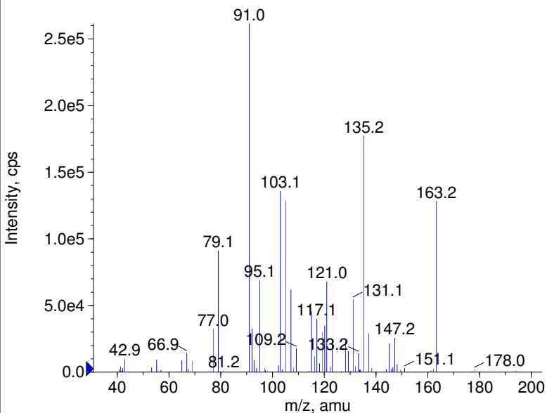
■ + DOM Prec(210.0) CE(50.0) RT(0.4)
