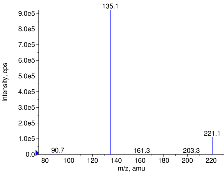
+ MDBP Prec(221.0) CE(50.0) RT(1.0)
