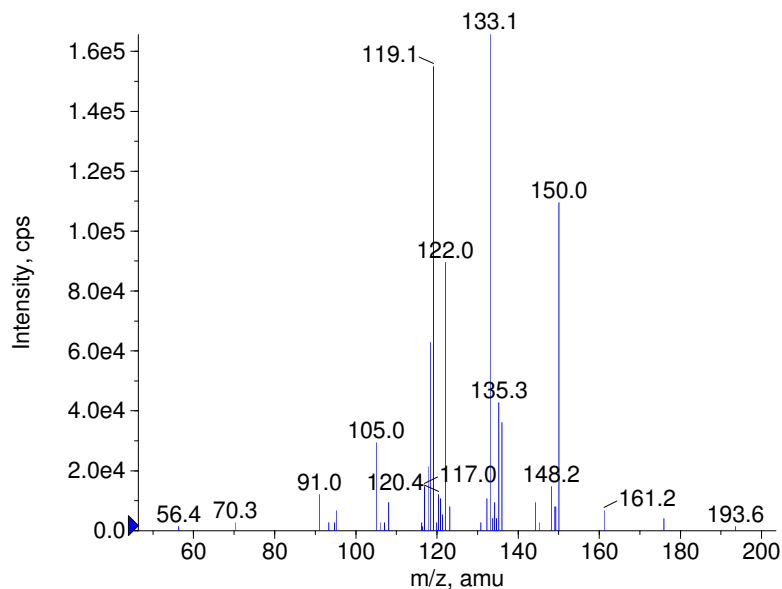
+ MeOPP Prec(193.0) CE(35.0) RT(0.5)
