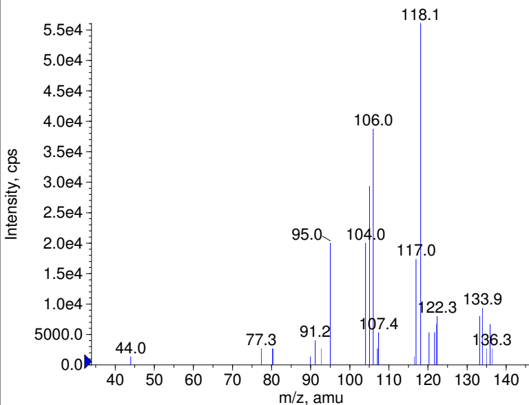
+ MeOPP Prec(193.0) CE(50.0) RT(0.5)
