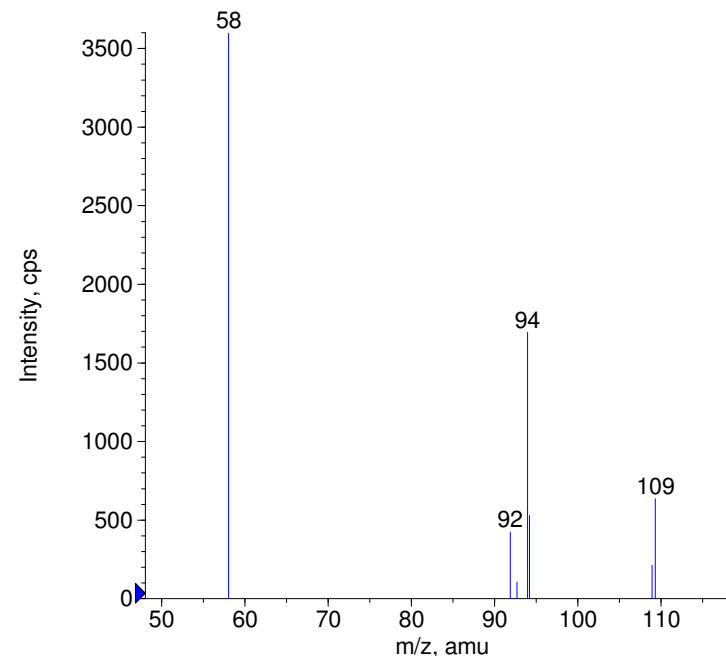
■ + Acipimox Prec(0.0) CE(0.0) RT(0.4)
