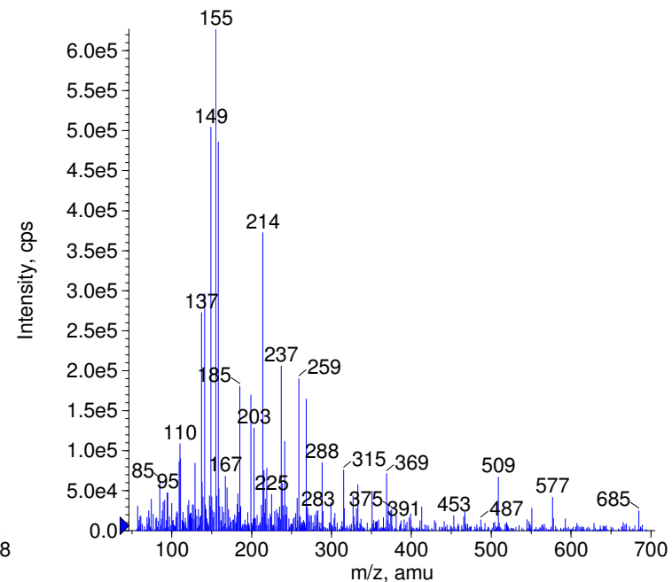
■ + Acipimox Prec(0.0) CE(0.0) RT(0.4)
