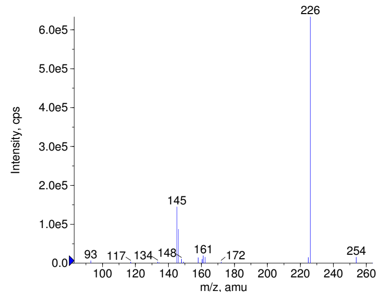
+ Actinoquinol Prec(254.0) CE(35.0) RT(1.1)
