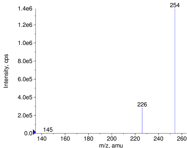
+ Actinoquinol Prec(254.0) CE(50.0) RT(1.2)
