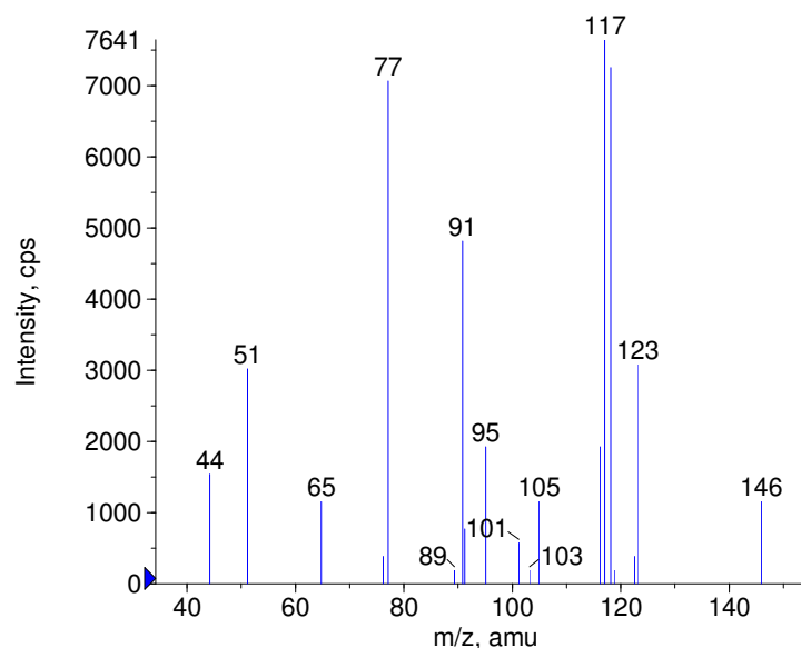
■ + Adrenalone Prec(182.0) CE(50.0) RT(0.3)
