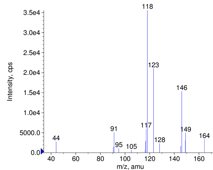
■ + Adrenalone Prec(182.0) CE(35.0) RT(0.2)
