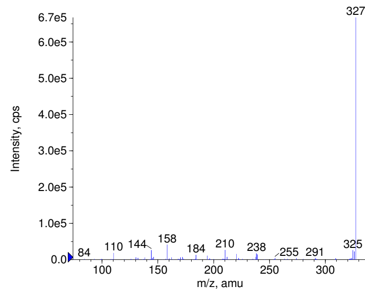
■ + Ajmaline Prec(327.0) CE(35.0) RT(0.2)
