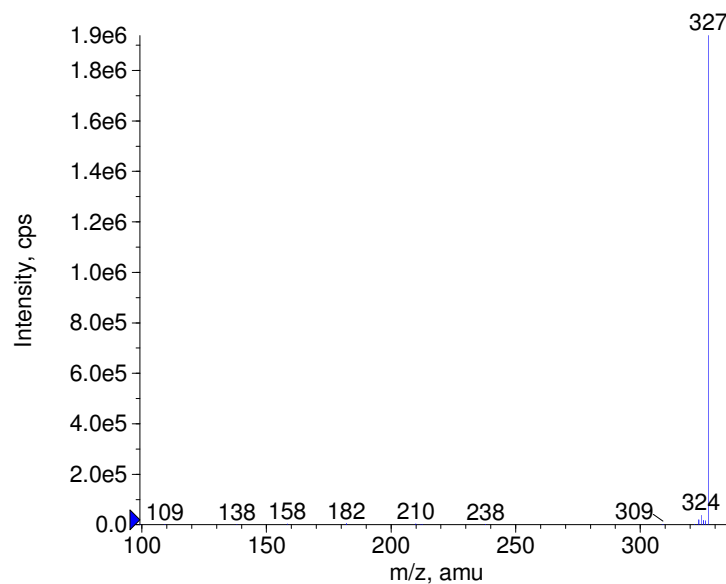
■ + Ajmaline Prec(327.0) CE(50.0) RT(0.3)
