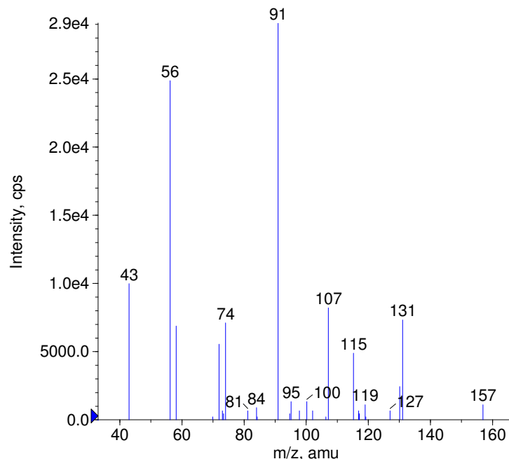
+ Alprenolol Prec(250.0) CE(50.0) RT(0.3)
