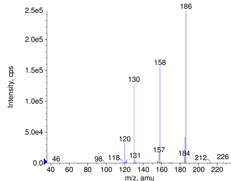
■ + Aminodantrolene Prec(285.0) CE(35.0) RT(2.6)
