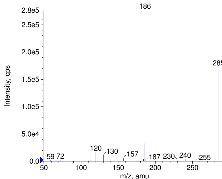
■ + Aminodantrolene Prec(285.0) CE(50.0) RT(2.6)
