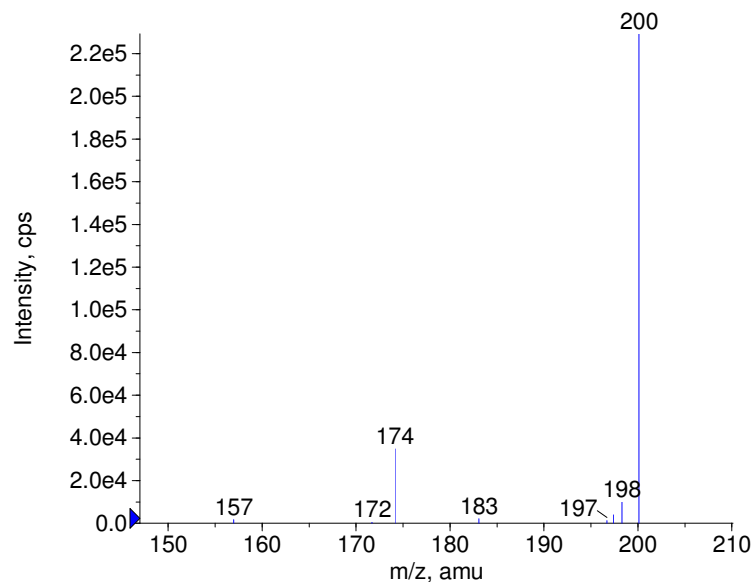
■ + Aminoquinuride Prec(373.0) CE(50.0) RT(0.3)
