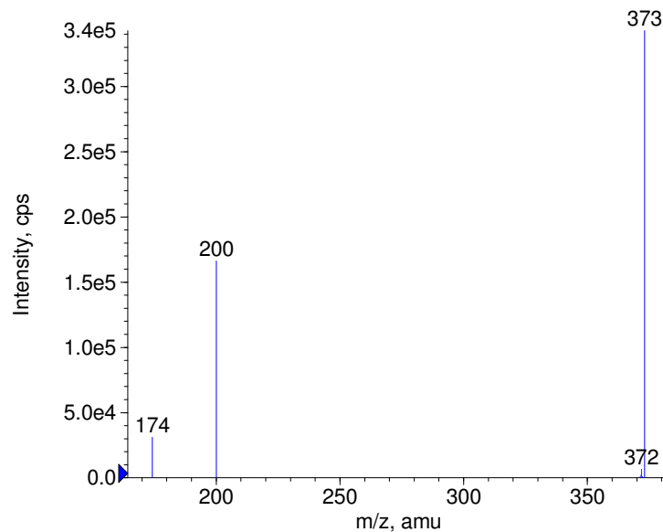
■ + Aminoquinuride Prec(373.0) CE(50.0) RT(0.3)
