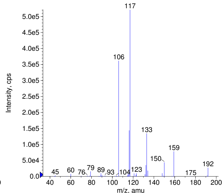
+ Amiphenazole Prec(0.0) CE(0.0) RT(0.4)
