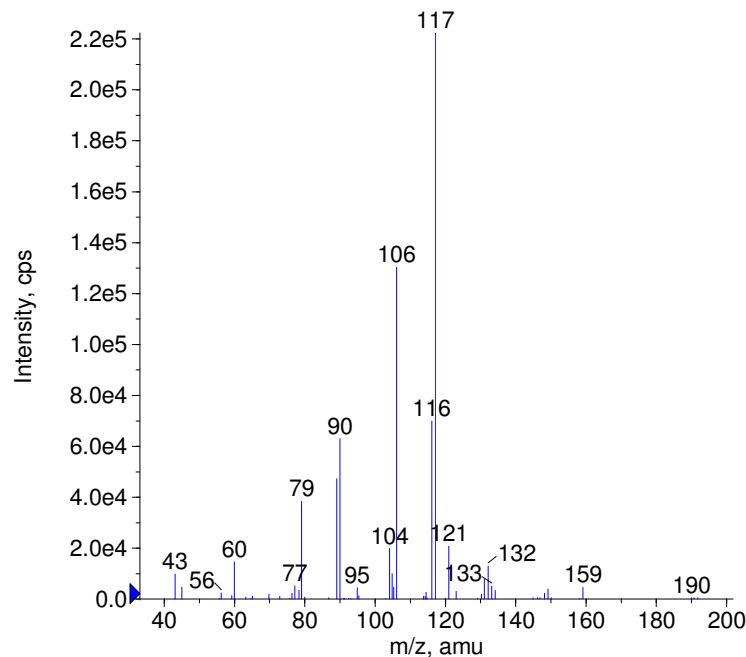
+ Amiphenazole Prec(192.0) CE(50.0) RT(0.3)
