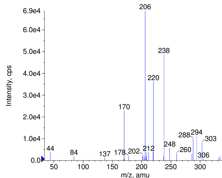
■ + Amlodipine Prec(409.0) CE(35.0) RT(0.2)
