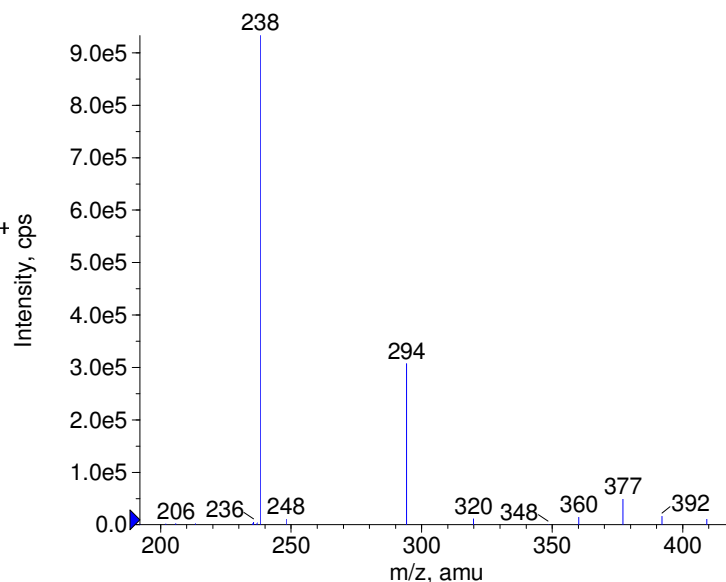
■ + Amlodipine Prec(409.0) CE(50.0) RT(0.2)
