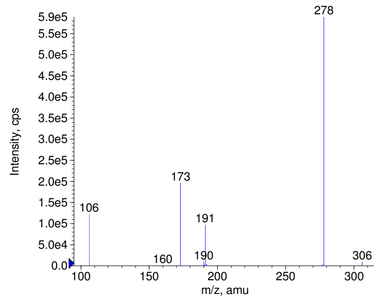
■ + Apalcillin Prec(522.0) CE(35.0) RT(2.9)
