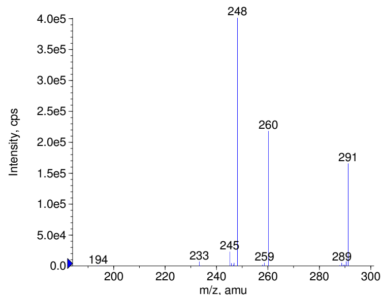
+ Azatadine Prec(291.0) CE(50.0) RT(0.3)
