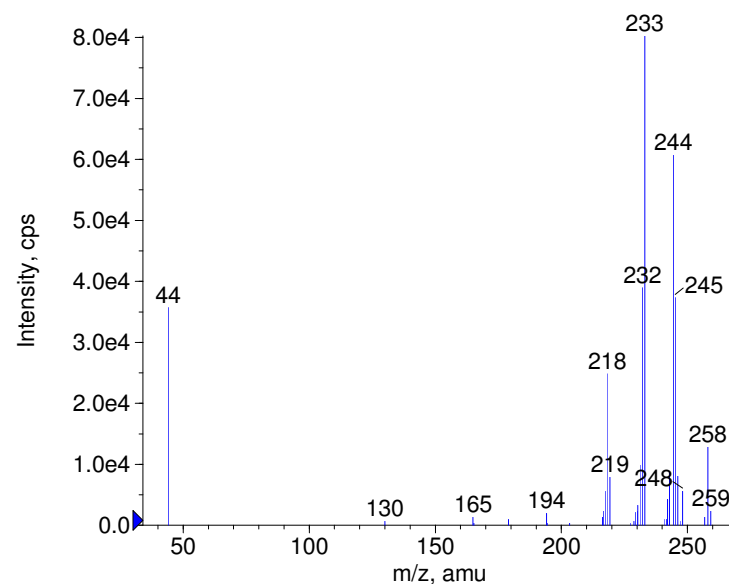
+ Azatadine Prec(291.0) CE(50.0) RT(0.3)
