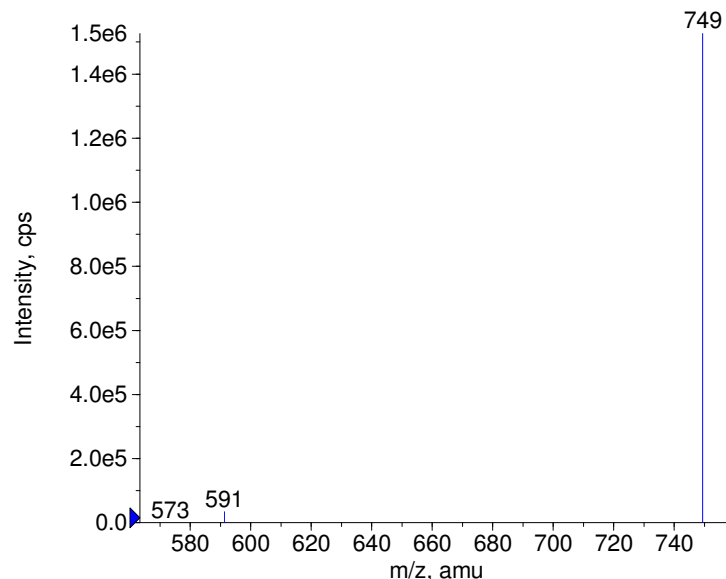
+ Azithromycin Prec(749.5) CE(50.0) RT(2.3)
