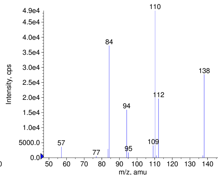
+ Azoluron Prec(231.0) CE(35.0) RT(0.2)
