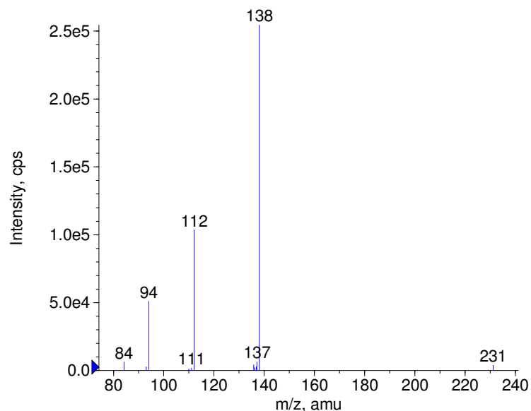
+ Azoluron Prec(231.0) CE(50.0) RT(0.3)
