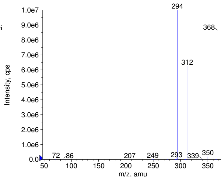
+ Bambuterol Prec(368.0) CE(50.0) RT(2.4)
