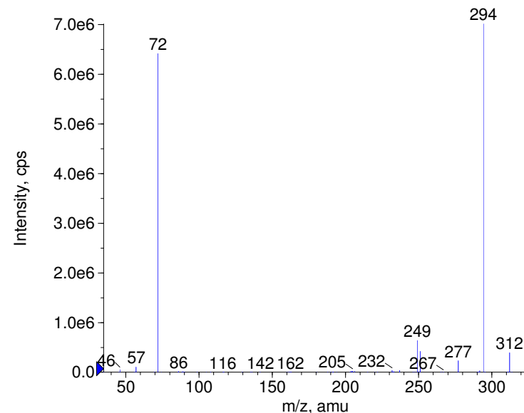
+ Bambuterol Prec(368.0) CE(35.0) RT(2.4)
