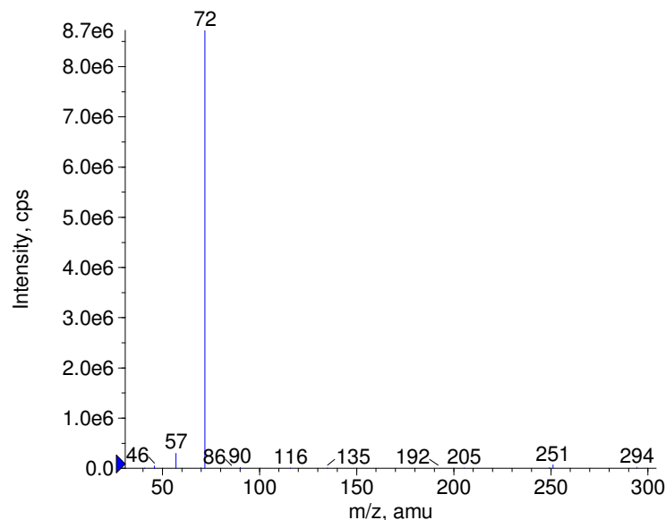
+ Bambuterol Prec(368.0) CE(50.0) RT(2.4)
