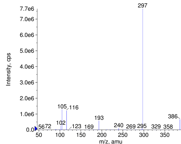
+ Bamifylline Prec(386.0) CE(35.0) RT(2.3)
