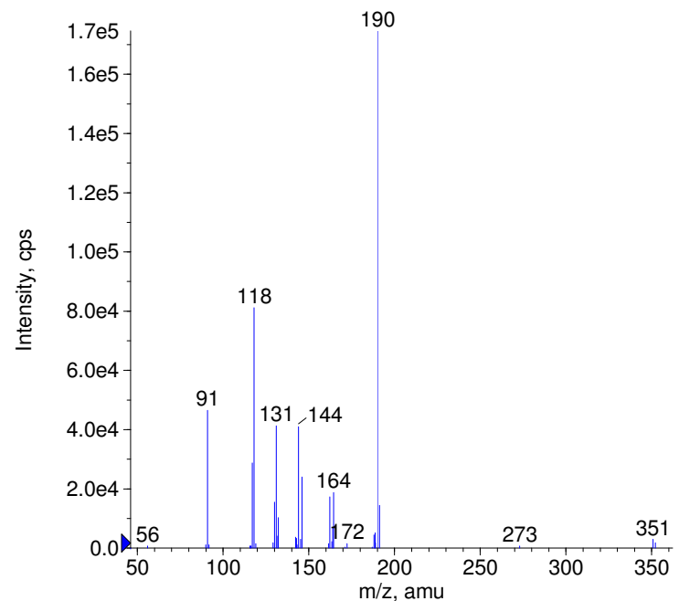
+ Benazeprilat Prec(397.0) CE(50.0) RT(0.3)
