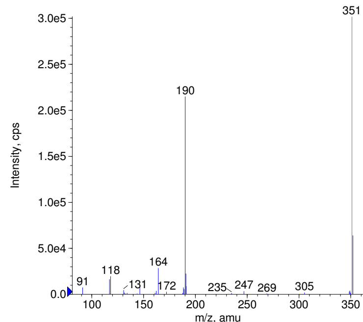
+ Benazeprilat Prec(0.0) CE(0.0) RT(0.4)
